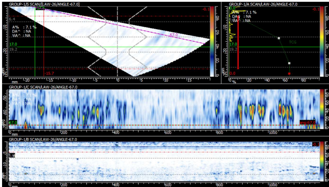
SPOOL-001 JUNTA-004
